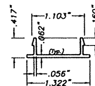
F SNAP CAP SCALE: 1/2" = 1"
