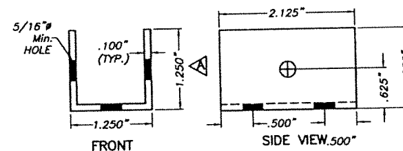
(N) H.V. STORM BAR CLIP
